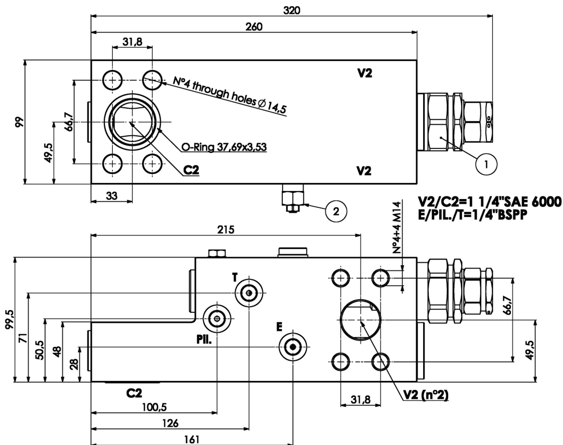
MOLLA VALVOLA (1) - SPRING VALVE (1)
